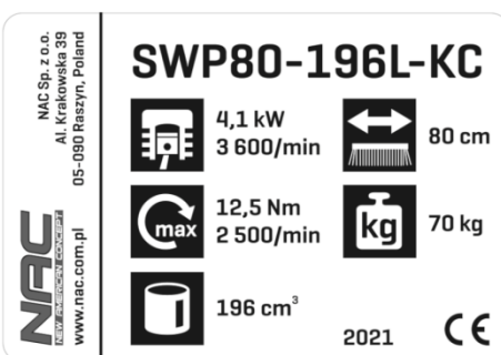
Tabliczka znamionowa
