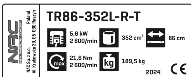
Tabliczka znamionowa
