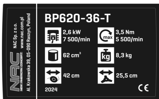
Tabliczka znamionowa
