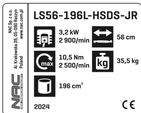
Tabliczka znamionowa
