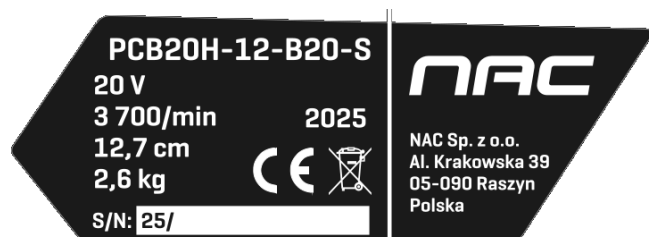
Tabliczka znamionowa
