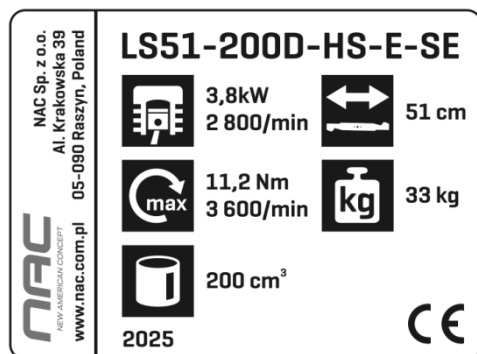
Tabliczka znamionowa
