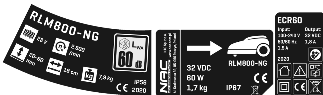
Tabliczka znamionowa znajdująca się na robocie
