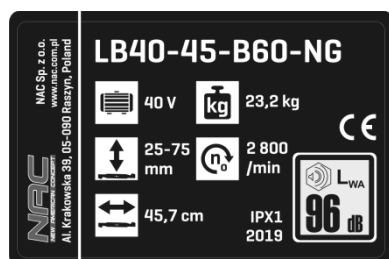
Tabliczka znamionowa
