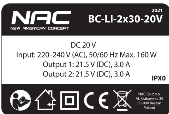
Tabliczka znamionowa
